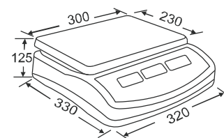
Dimension(mm)
